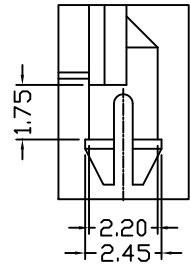
DETAIL A 2:1
